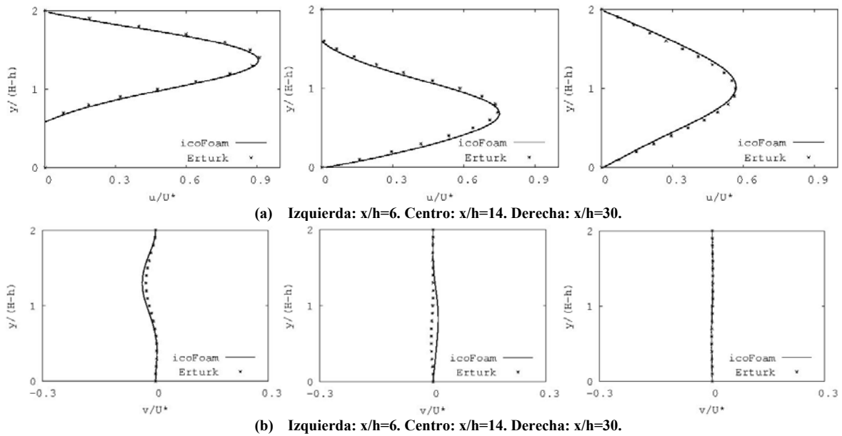
Figura 4. Perfiles de velocidad adimensional en diferentes ubicaciones del canal de entrada a partir del escalón. T=400 . L_1=20 . L_2=300 . Arriba: valores de velocidad horizontal, u . Abajo: valores de velocidad vertical, v .
