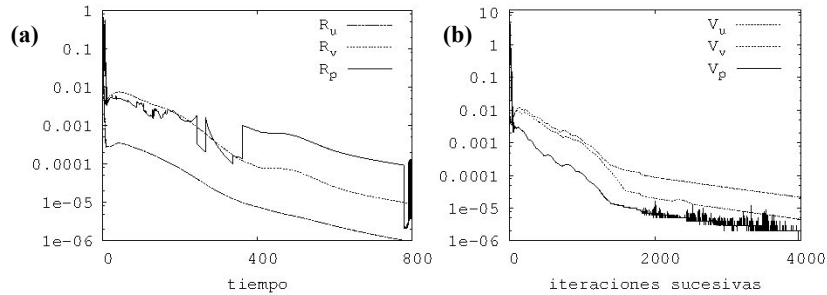
Figura 3. Evolución de V\phi y R\phi durante 800 segundos de simulación. L_1 = 20 , L_2 = 300 .
